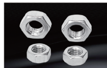
六角重型螺母 HEX HEAVY NUT 材质 Material: SUS304 A2,SUS316 A4 规格 Size: M6-M45 3/8" -1-1/4" 标准 Standard: DIN,ASME,ANSI
