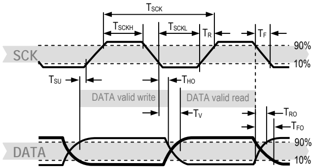
图 11: 时序图,缩写词在表 3 有注释。加重的 DATA 线由传感器控制,普通的 DATA 线由单片机控制.有效时间依据 SCK 的时序。请注意 数据读取的有效时间为前一个切换的下降沿。
