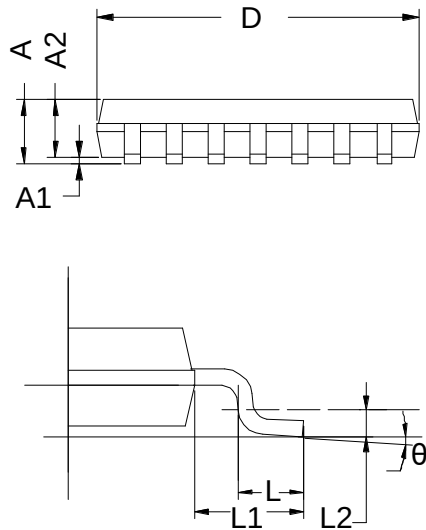
TSSOP14
