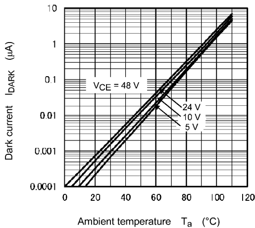
Fig. 11.11 I_{DARK} - T_a
