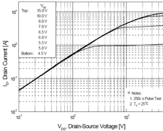
图1 输出特性曲线, Tc=25°C
