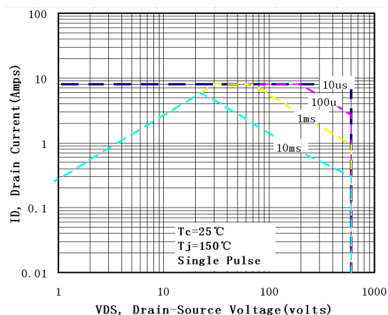
图 6-2 2N60(TO-220F)
