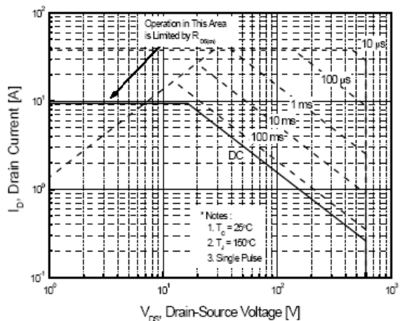
图 6-1 10N65(TO-220)
