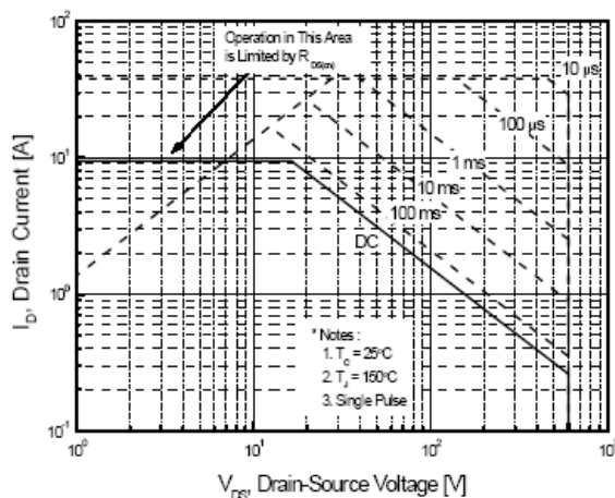
图 6-1 10N65(TO-220F)
