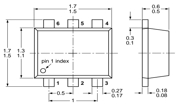
PESDxL5UV (SOT666)
