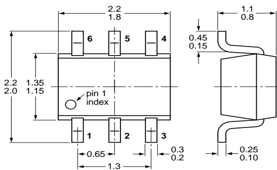
PESDxL5UV (SOT666)
