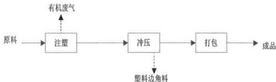
图 2-1 本项目工艺流程及产污环节
