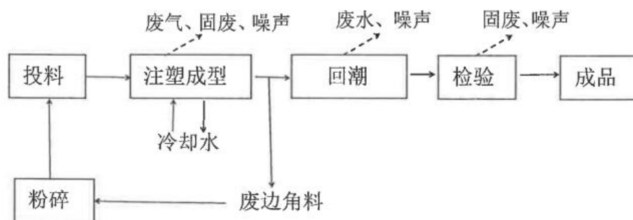
图 2-1 本项目工艺流程及产污环节
